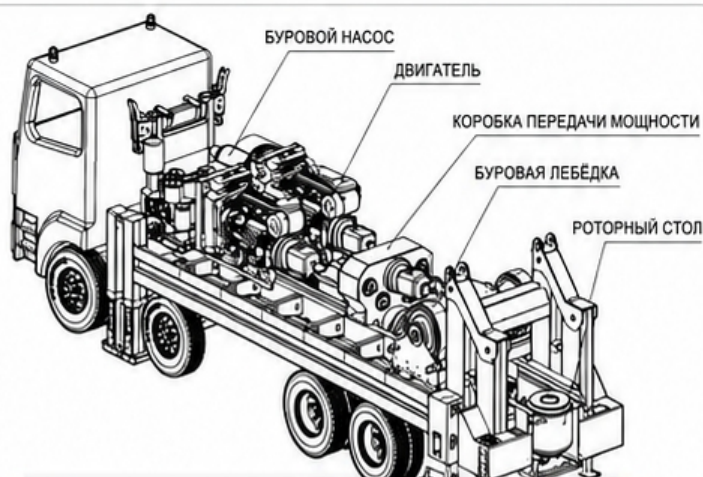
БУРОВАЯ УСТАНОВКА НА ГРУЗОВОМ ШАССИ
