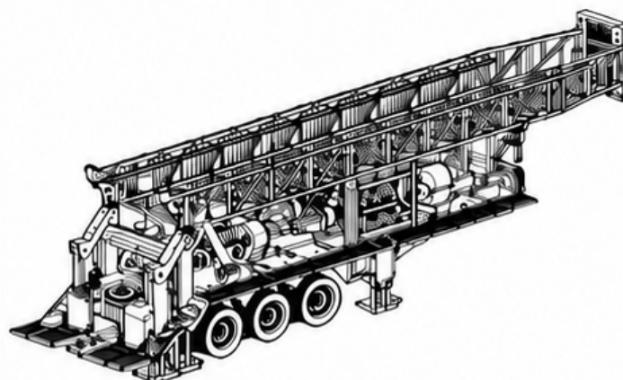
БУРОВАЯ УСТАНОВКА НА ПРИЦЕПЕ
